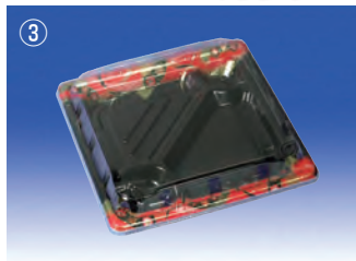
なごみ膳23-23-1本体 ●サイズ：225×225×23 なごみ膳23-23蓋 (ユーガード) 53333 ●サイズ：229×229×34
